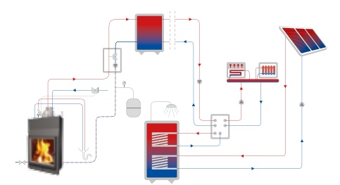
mit Anbindung an die Zentralheizung
