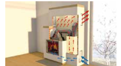
Kombi-Speicher-Kamin
